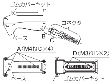
形番：HE9Z-GP15
