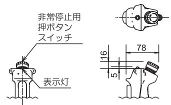
形番：HE2G-2□HE-P*-0
