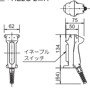
形番：HE2G-2□HE-L-K
