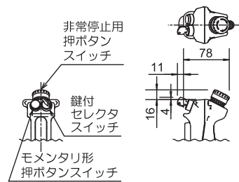
形番：HE2G-2□HE-L-K
