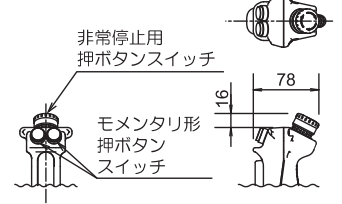
形番：HE2G-2□HE-L-L
