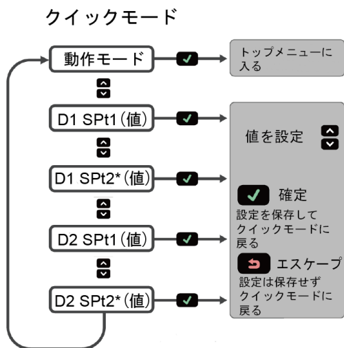
図 6 クイックモードの階層図 (ウインドウモードの場合)
