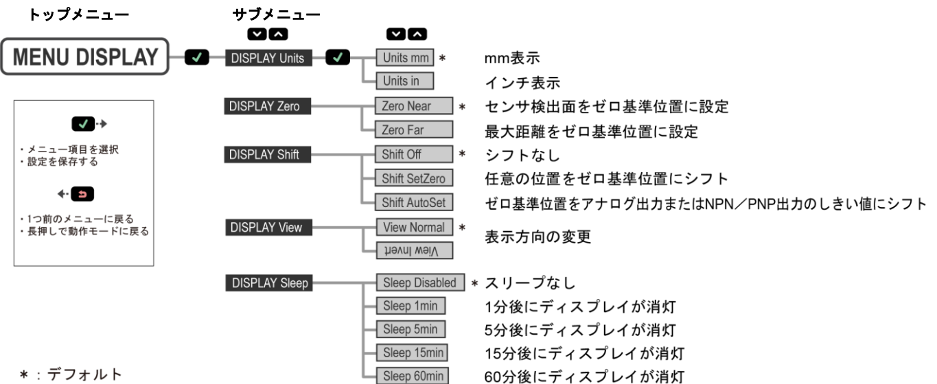
図 8-4 ディスプレイメニューの階層図
