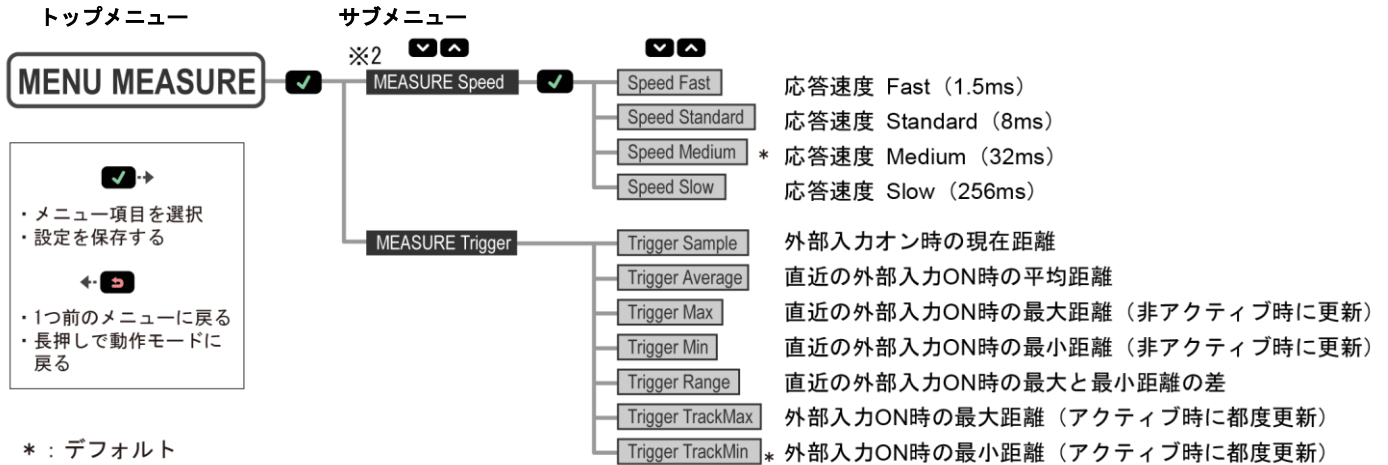
図 8-3 測定メニューの階層図
