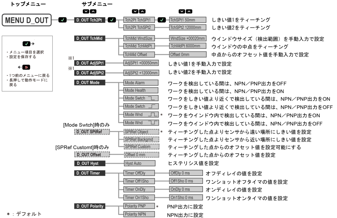
図 8-1 NPN/PNP 出力メニューの階層図
