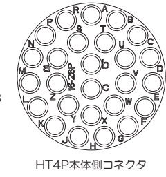
HT4P本体側コネクタ
