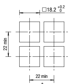
Square (LB7S/LB7MS)
