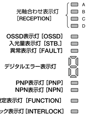
受光器側の表示灯部
