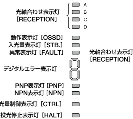
投光器側の表示灯部
