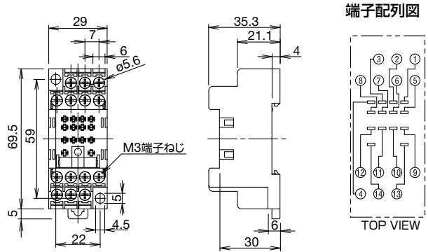
端子配列図
