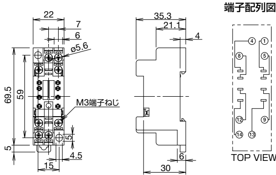
端子配列図
