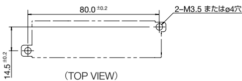
(取付穴加工寸法)
