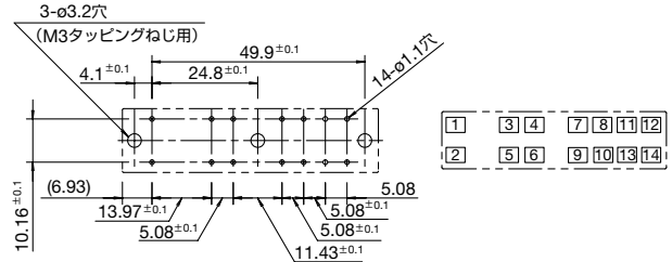
[プリント基板加工図・端子配列 (BOTTOM VIEW)]
