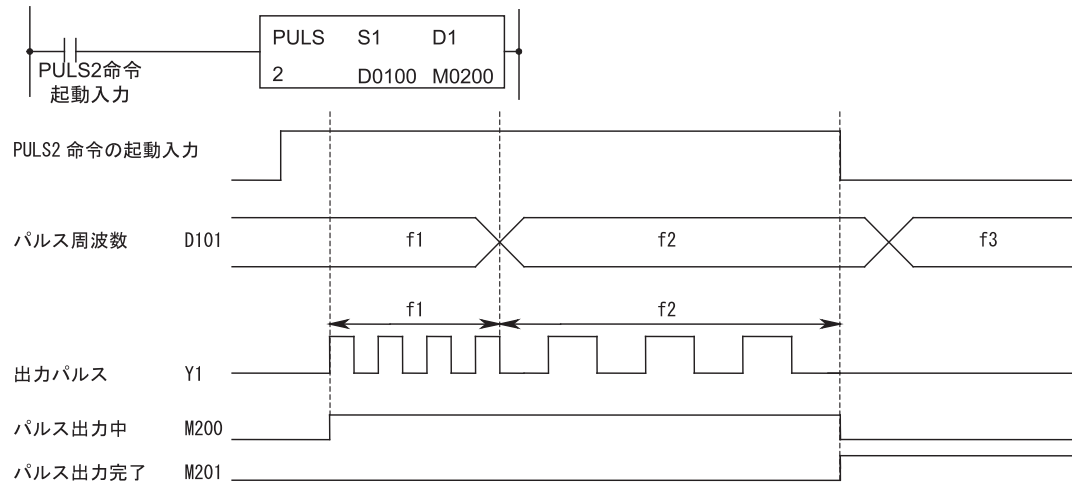
f1、f2、f3 はパルス周波数
