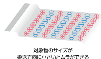
AC方式 (一本の針から+または-イオンを交互に発生)
