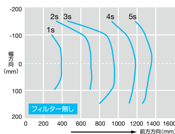
除電領域 — 除電時間特性図（*3）
