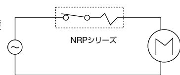
モータのコイル保護
