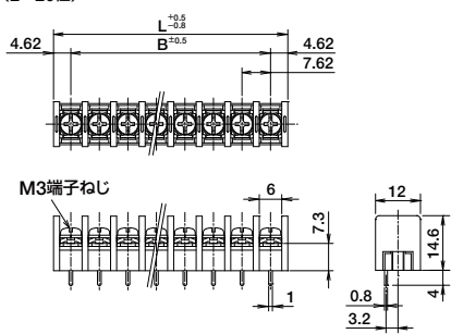
外形寸法図 (2~20極) (単位：mm)
