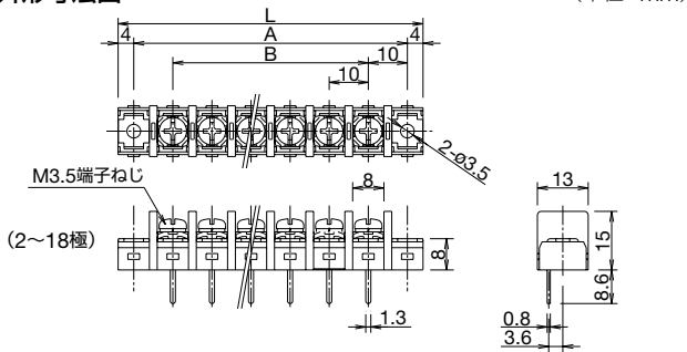
外形寸法図
