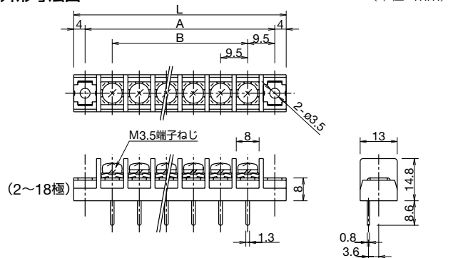
外形寸法図
