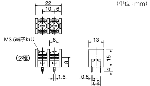
外形寸法図
