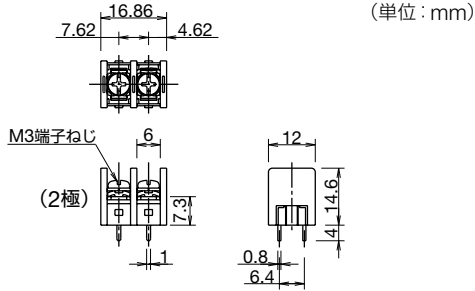
外形寸法図
