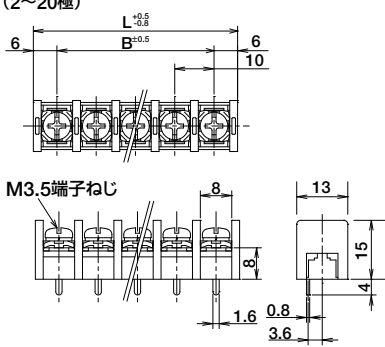
外形寸法図 (2~20極) (単位：mm)
