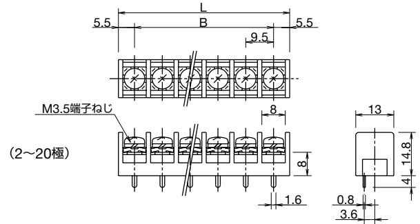
外形寸法図 (2~20極) (単位：mm)
