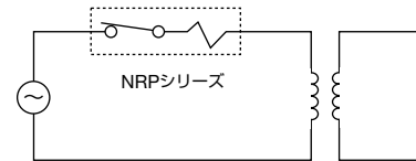
トランス保護例 トランス1次側保護
