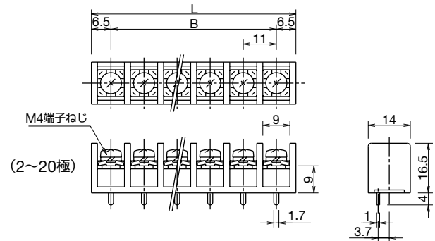
外形寸法図 (2~20極) (単位：mm)
