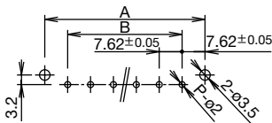
外形寸法図
