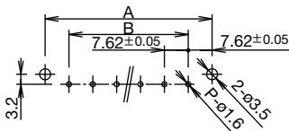
外形寸法図 (単位：mm)
