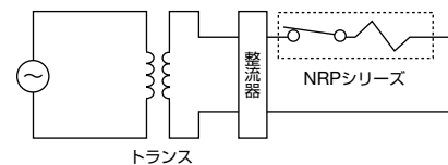
整流器保護例
