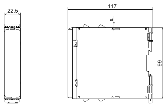
HR6S-BAC形
