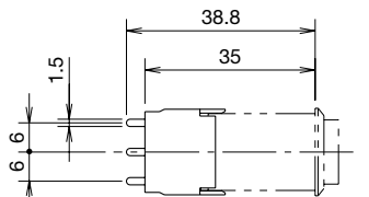
プリント基板用端子形ソケット (形番: MA9Z-C3V)
