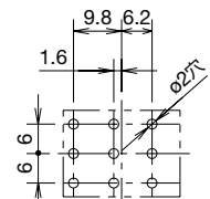
プリント基板加工図 (BOTTOM VIEW)
