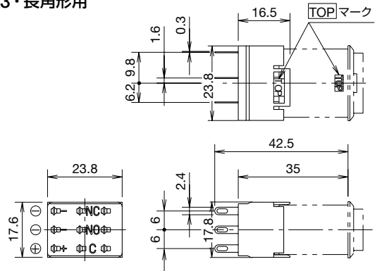
溶ダ端子形ソケット (形番: MA9Z-C3)
