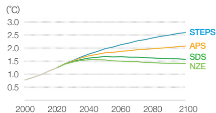
WEOシナリオ別地表温度平均値上昇推移
