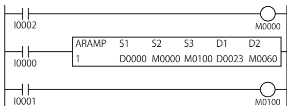
ラダー図
