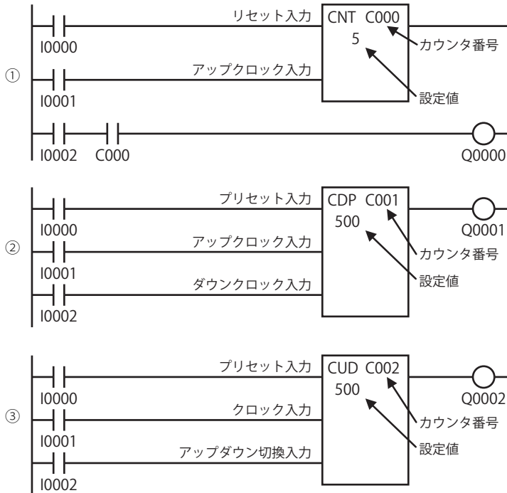
ラダー図
