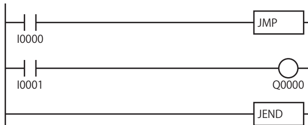
ラダー図
