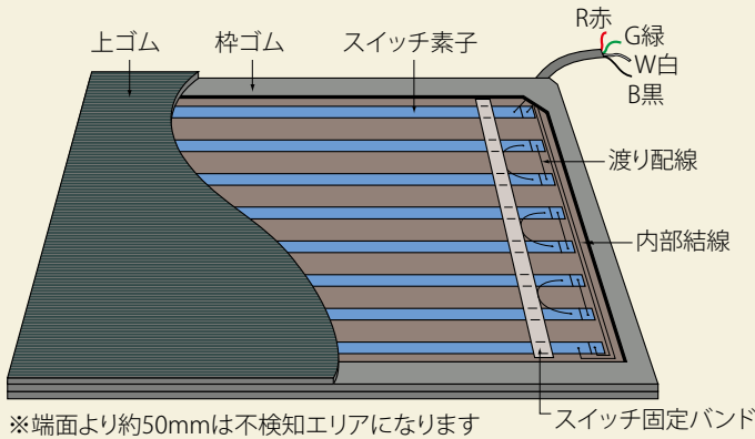
【構造図】
