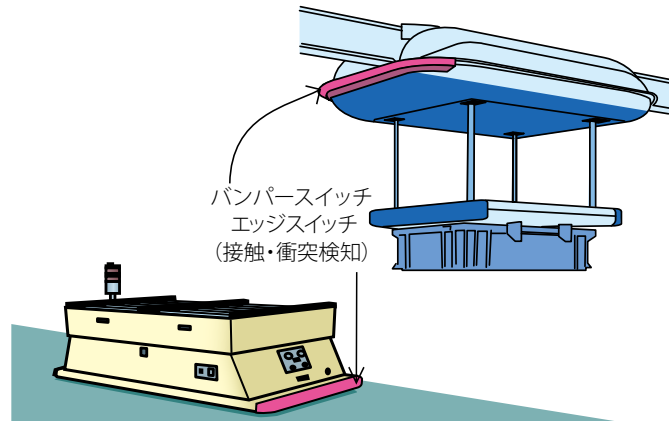
コンベア
