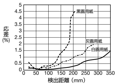
●色(200×200mm画用紙)、材質-検出距離特性(200mm設定時)
