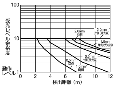
● 平行移動特性(0.5mm縦スリット装着時)
