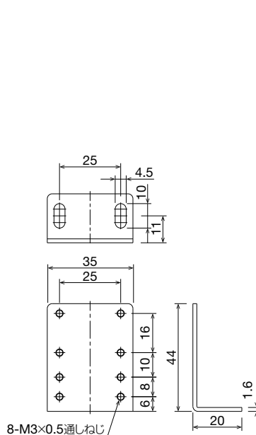
(材質:SPCC)
