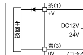
(コネクタピン配置)
