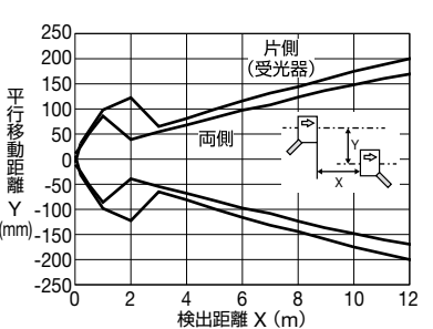
● 平行移動特性(2.0mm丸スリット装着時)
