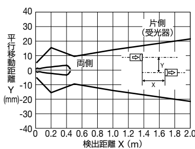
● 平行移動特性(0.5mm丸スリット装着時)
