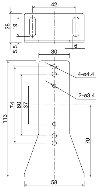
(材質:SPCC)
