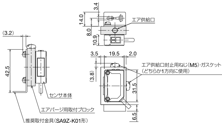
取付金具装着時
