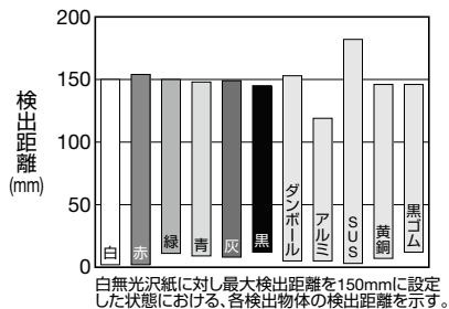
●色(100x100mm 無光沢紙)、材質—検出距離特性(150mm設定時)
