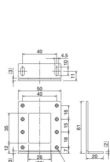
(材質:SPCC)
