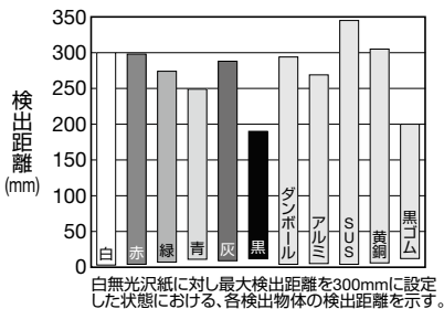
●色(100x100mm 無光沢紙)、材質—検出距離特性(300mm設定時)
