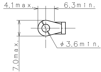
適合圧着端子寸法
