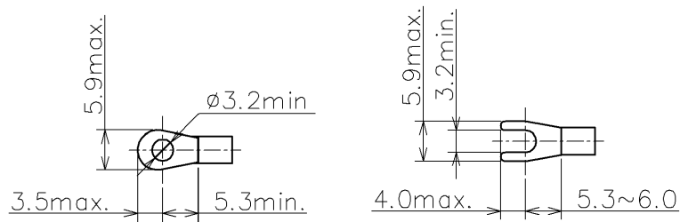
適合圧着端子寸法
