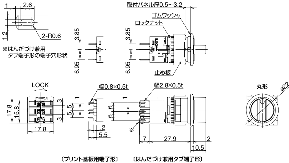
〔プリント基板用端子形〕
