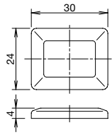
長角形ユニット用 (LB9Z-D8形)
