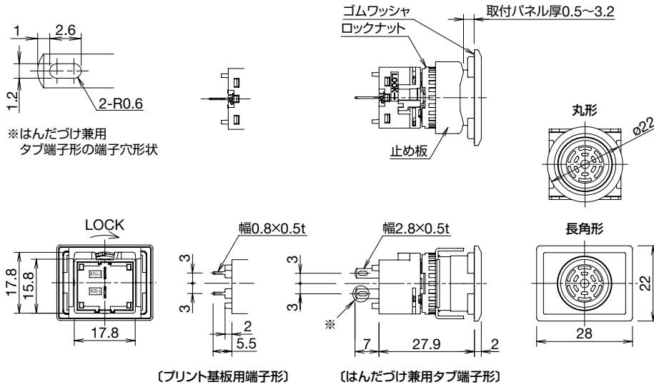
〔プリント基板用端子形〕
