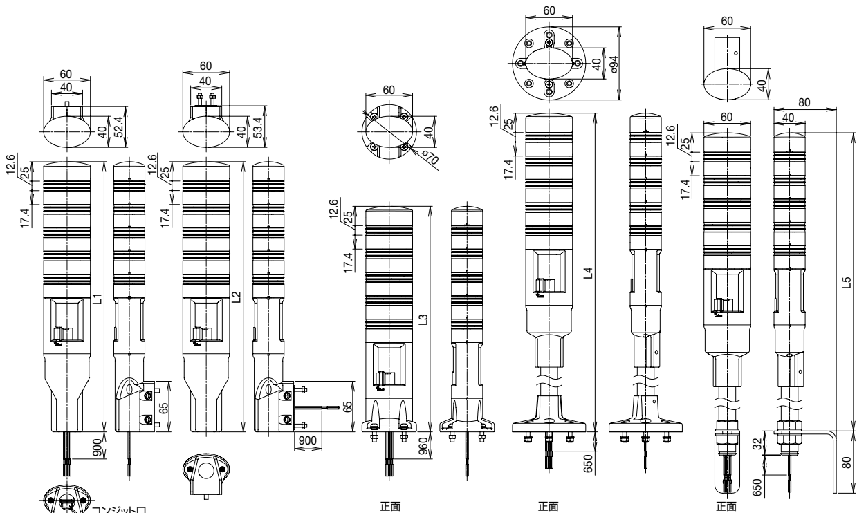
寸法一覧表
