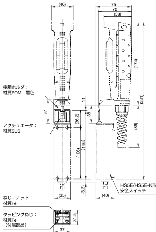
HE1G-L形グリップスイッチおよび HS5E/HS5E-K形安全スイッチと組み合せた状態
