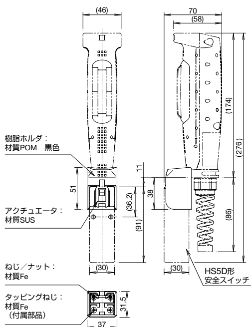
HE1G-L形グリップスイッチおよび HS5D形安全スイッチと組み合せた状態
