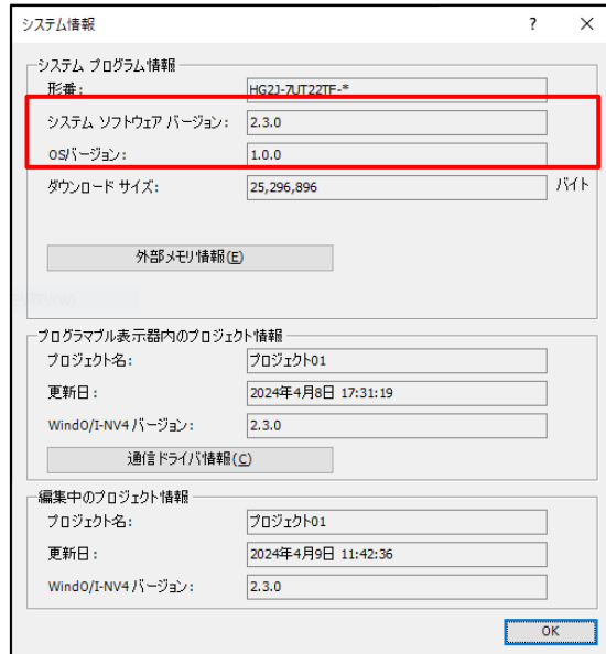
図-1：[システム情報]ダイアログボックス
