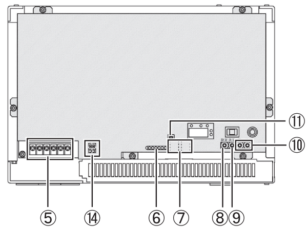
正面カバーを外した状態
